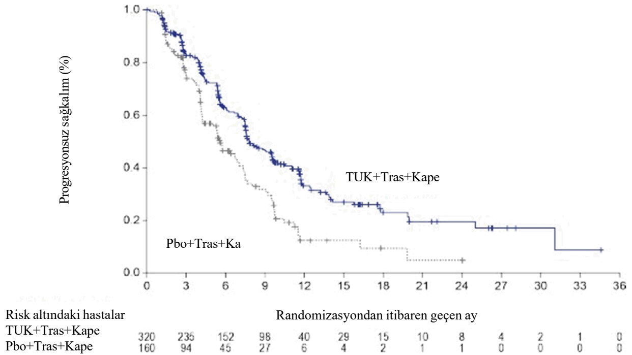
Şekil 1. (KBMİ'ye göre) progresyonsuz sağkalıma ait Kaplan-Meier eğrileri
